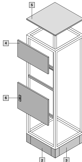
Комплектующие шкафа
