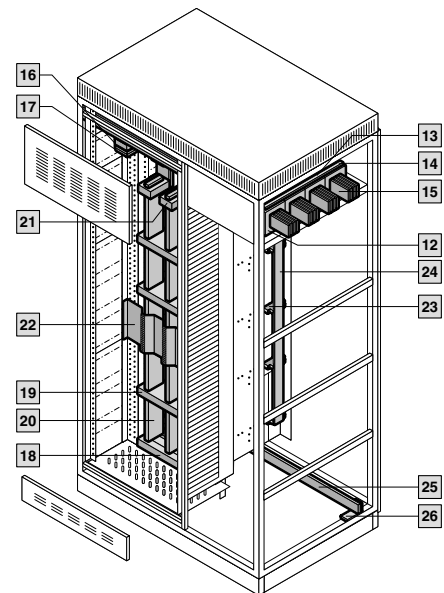
Комплектующие шкафа
