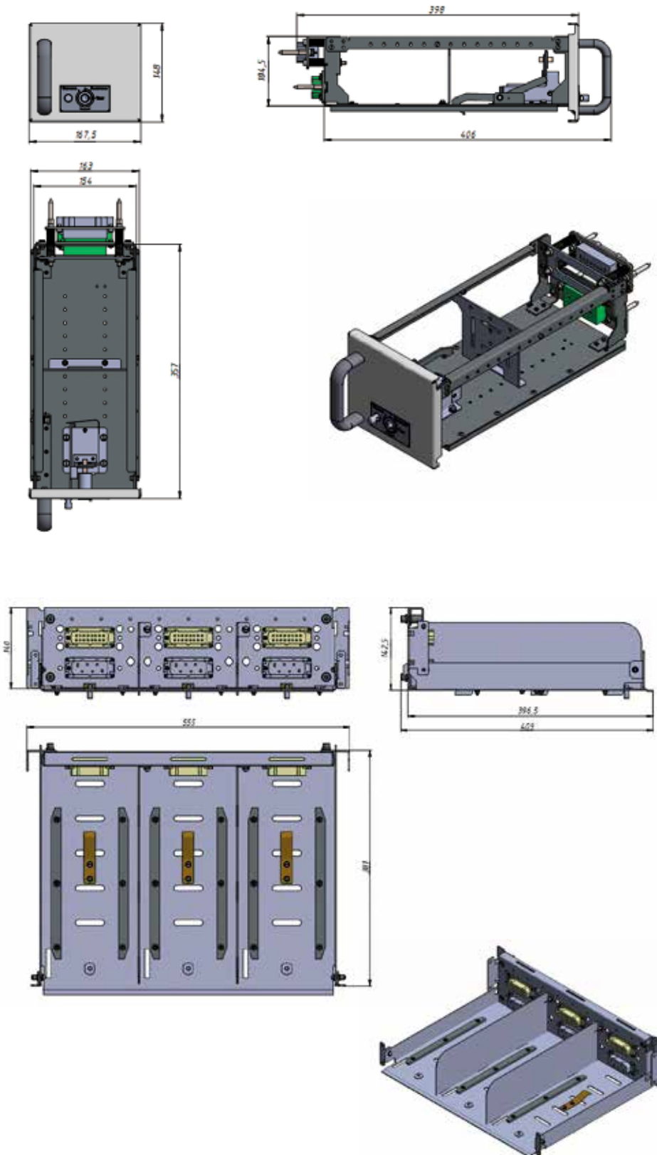
Типоразмеры 1_3
