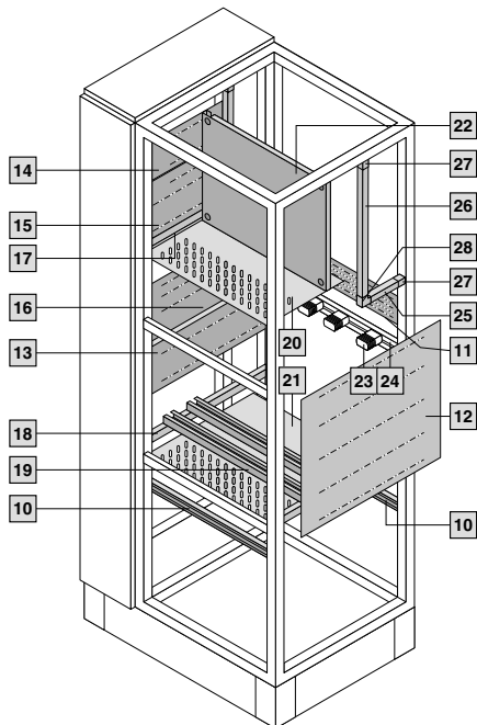
Оборудование секции
