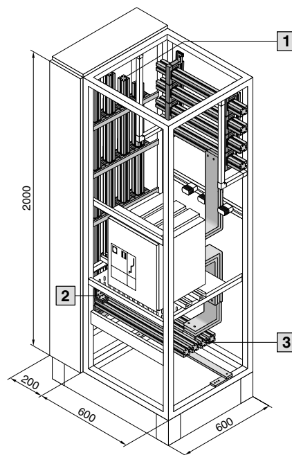
Шинные системы
