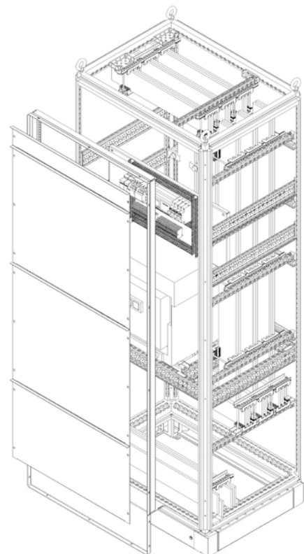
Пластронная система
