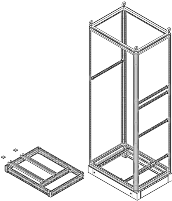
Система профилей
