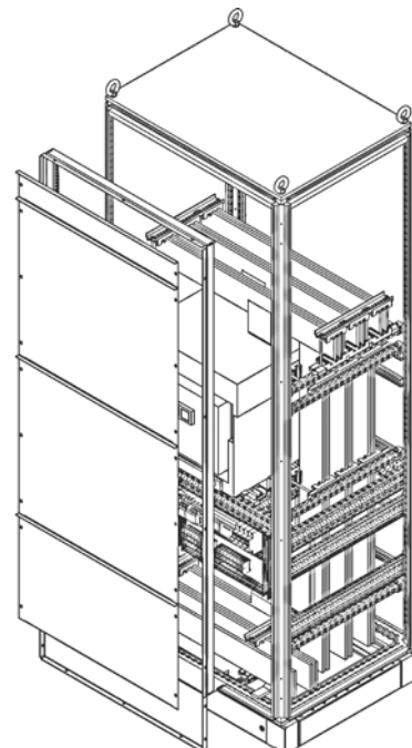
Пластронная система
