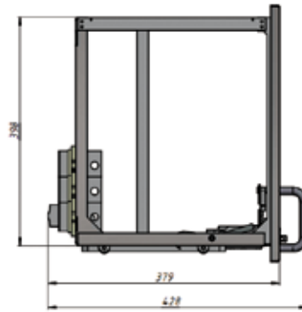
Типоразмеры 3_1
