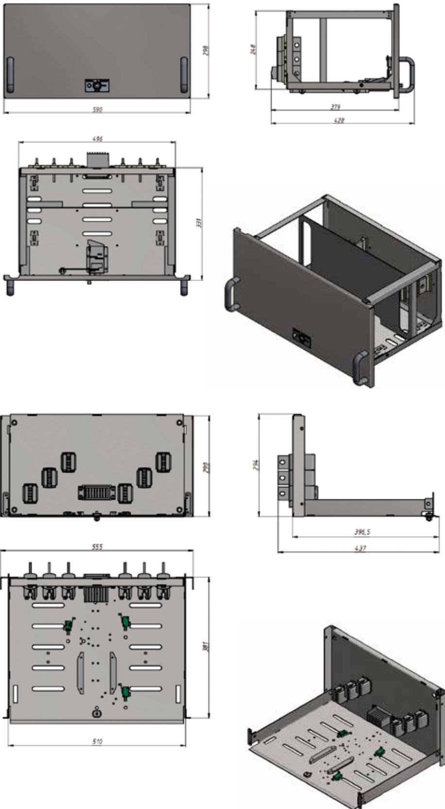
Типоразмеры 2_1
