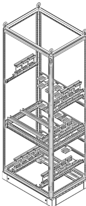
Шинодержатели
