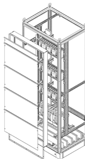
Платорная система
