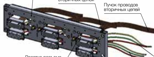
Розетка разъема вторичных цепей
