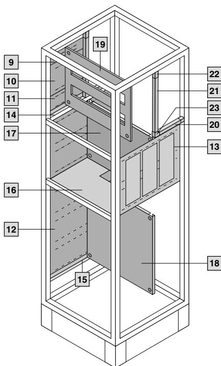
Оборудование секции
