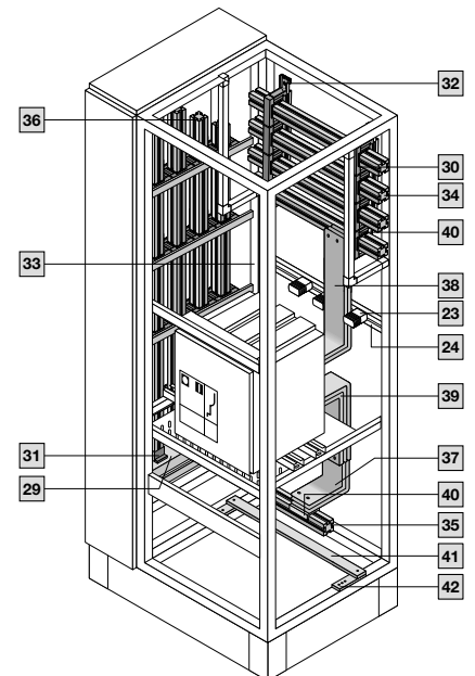
Шинные системы
