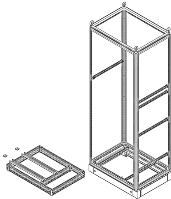
Система профилей
