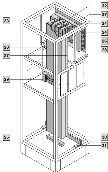
Шинные системы
